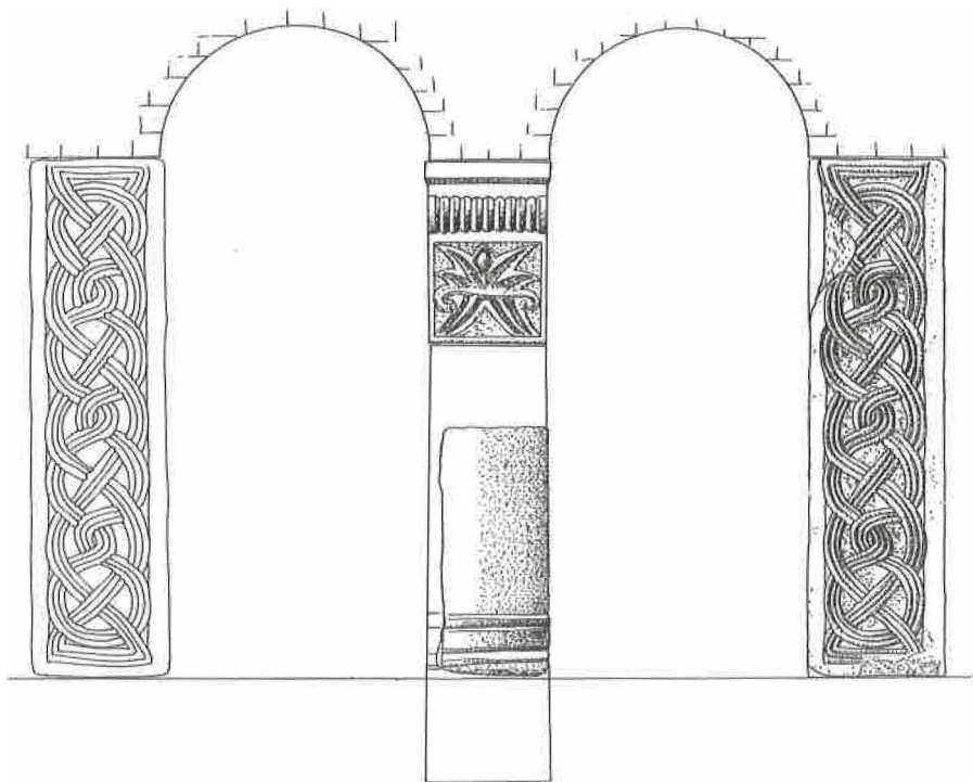
Sl. 26. Galovac, Crkvina - grafički prikaz pretpostavljenog izvornog izgleda dvojnog prozora (bifore) druge predromaničke faze.
