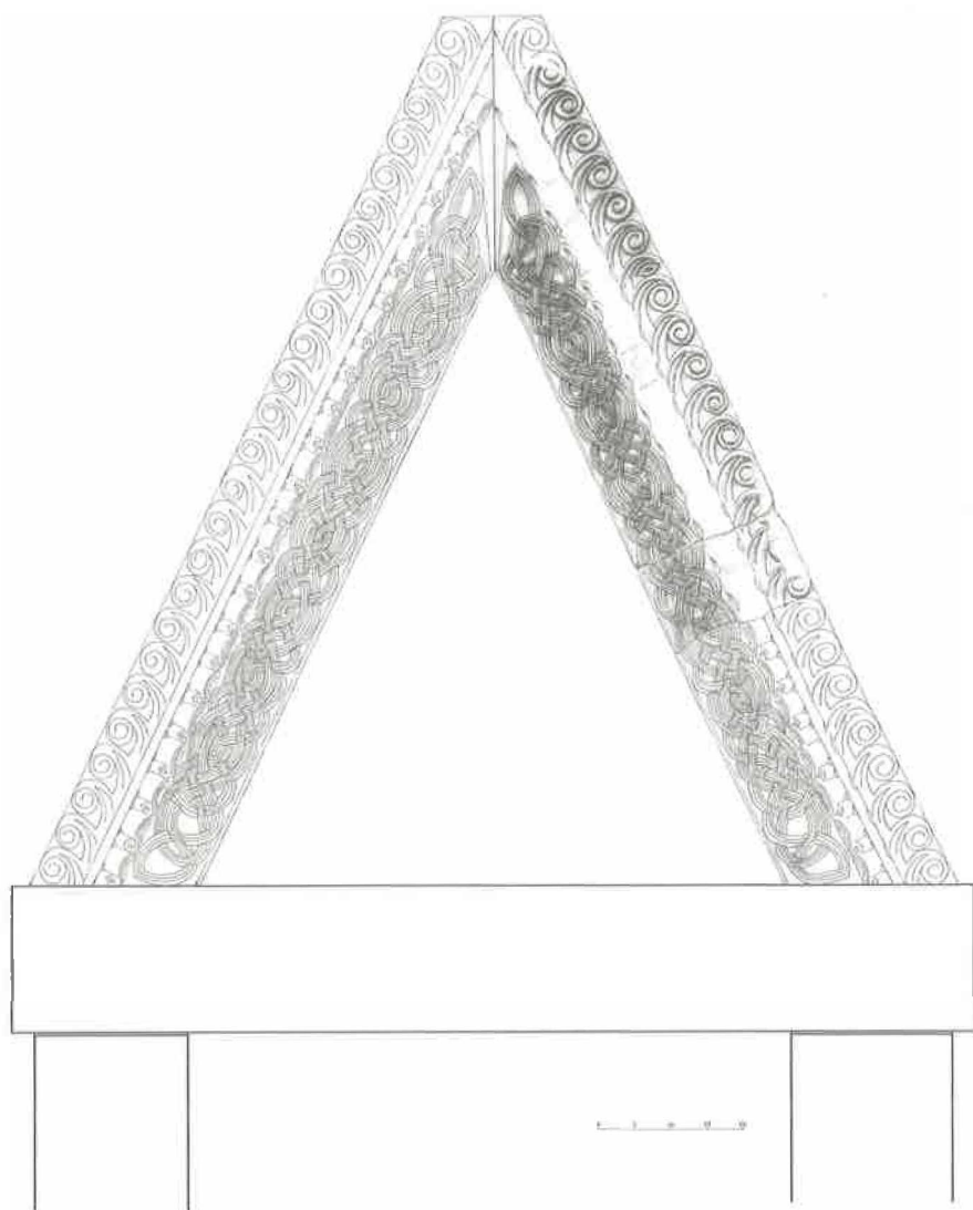
Sl. 24. Galovac, Crkvina - grafički prikaz pretpostavljenog izvornog izgleda ukrasne oplata vrata druge predromaničke faze.
